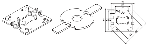
快速连接件/quick plug A3067
