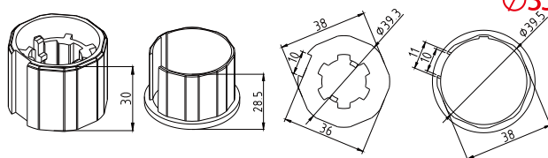
皇冠驱动轮A2308 Ø35
