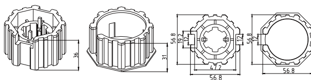
皇冠驱动轮A2407 Ø45
