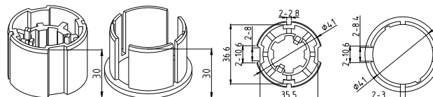
皇冠驱动轮A2308 Ø35
