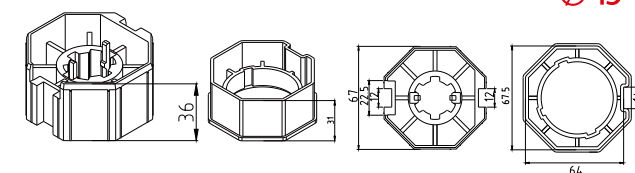
皇冠驱动轮A2408 Ø45
