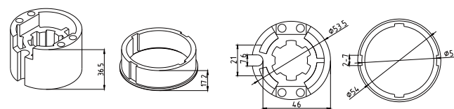
皇冠驱动轮A2406 Ø45
