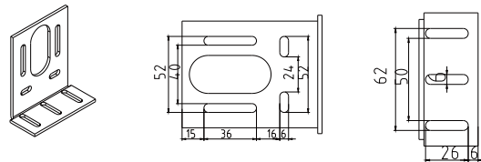
尾塞支架/bracket A3028
