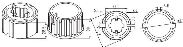
皇冠驱动轮A2309 Ø35
