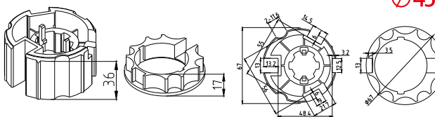
皇冠驱动轮A2408 Ø45
