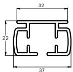
A型轨道 (Track A system)
